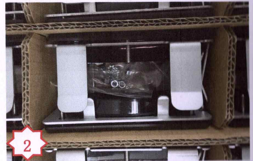
图二，将 1 袋装好的螺母垫圈和 2PCS PA984 如图装入单元格中。
